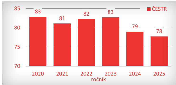
Graf 4 – Průměrné lineární skóre 0–4 % u farem v kategorii Čestř v jednotlivých ročních soutěže
