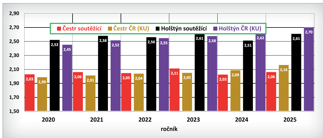
Graf 11 – Vývoj průměrného obsahu tuku a bílkovin u soutěžících a v kontrole mléčné užitkovosti v ČR
