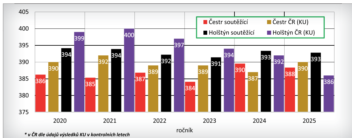
Graf 8 – Délka mezidobí u soutěžících a u podniků zařazených do kontroly mléčné užitkovosti v ČR
