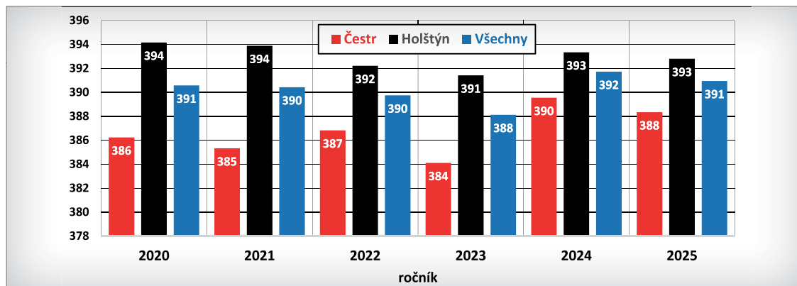
Graf 7 – Průměrná délka mezidobí u soutěžících podle kategorií v jednotlivých ročních soutěže
