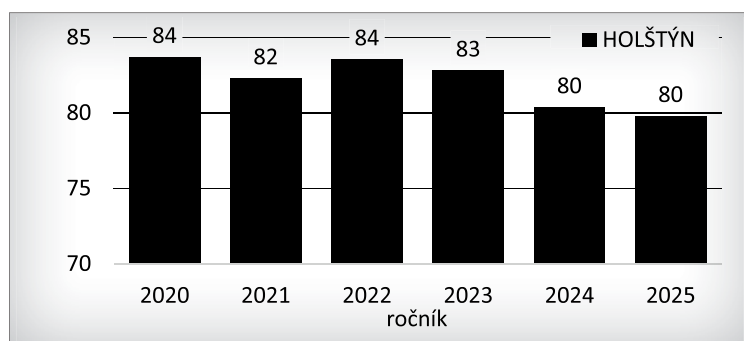
Graf 5 – Průměrné lineární skóre 0–4 % u farem v kategorii Holštýn v jednotlivých ročních soutěže
