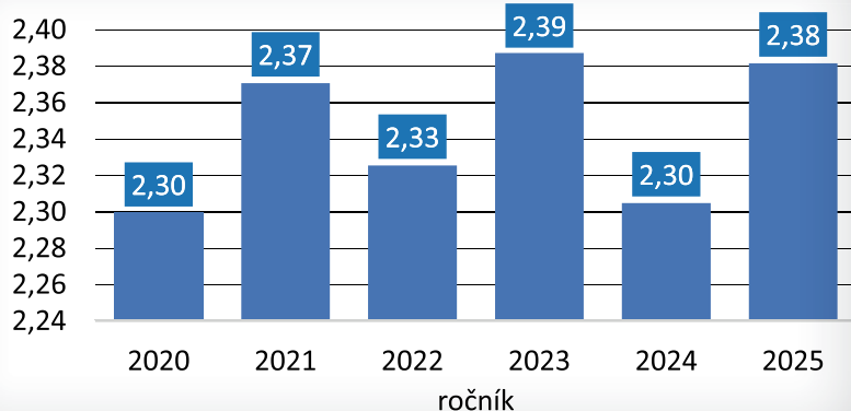
Graf 10 – Vývoj obsahu tuku a bílkovin (v kg) u všech soutěžících
