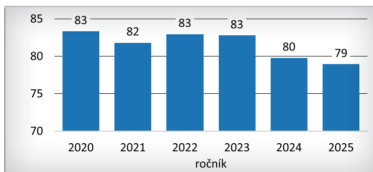
Graf 6 – Průměrné lineární skóre 0–4 % u všech soutěžních farem v jednotlivých ročních soutěže
