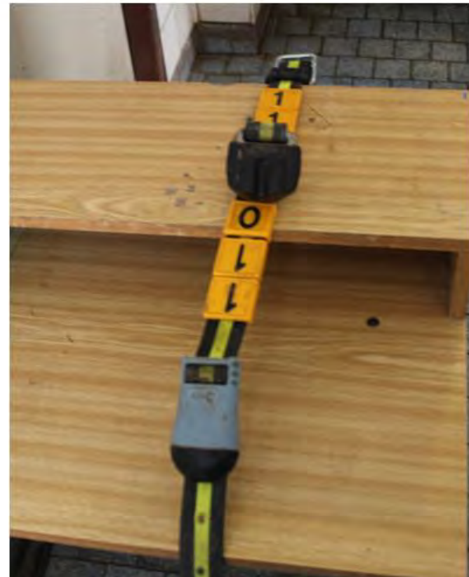
Tlumačov – obojky SCR pro monitoring žvýkání a pohybu
